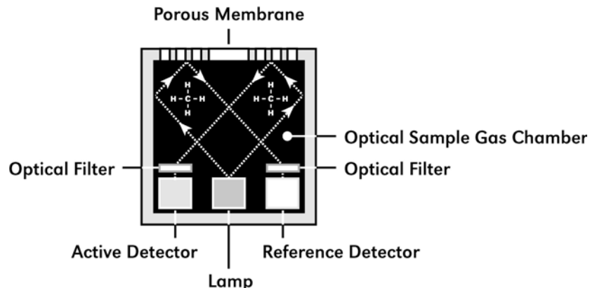
Figure 1 Construcción del Sensor
