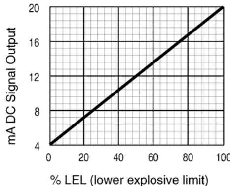
Figura 3 Curva de Respuesta
