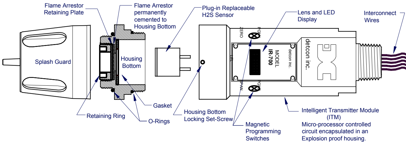
Figure 5 Desglose del Armado del Sensor
