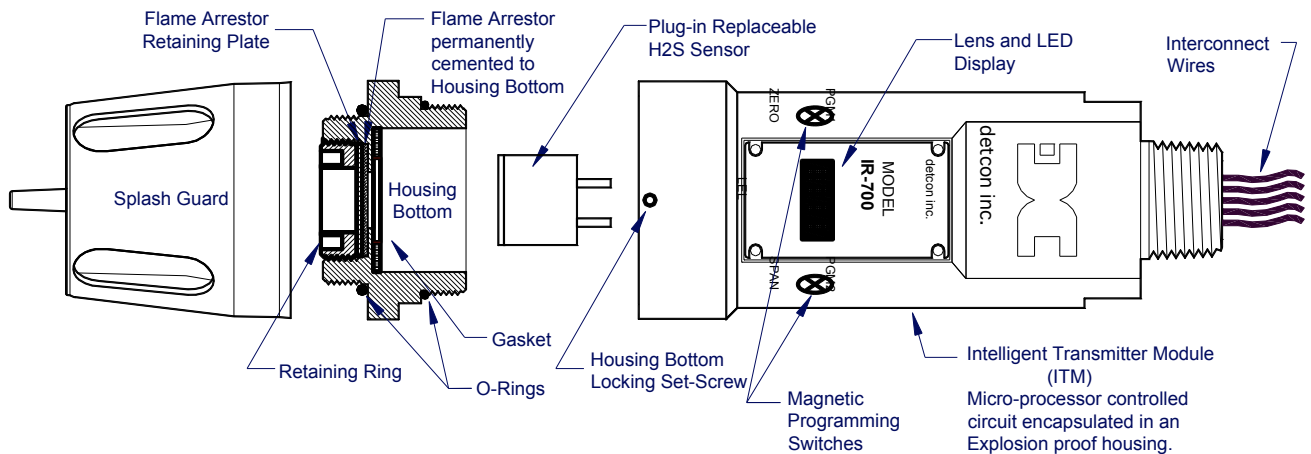
Figure 14 Ensamble del Sensor
